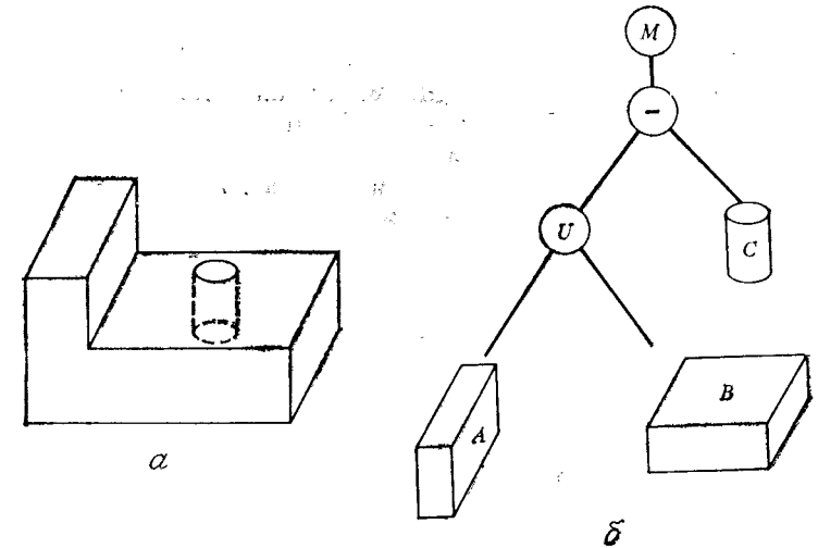
Рис. 10.19. Пространственная геометрия воспроизведения объектов. Атрибуты A и B : длина, ширина, высота. Атрибуты C : радиус, высота. Набор операторов-связей: U — объединение, \cap — пересечение, - — разность.
