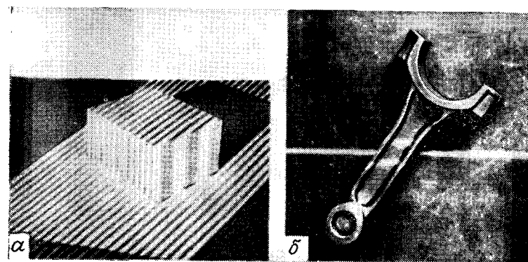
Рис. 7.9. Два примера структурного освещения [250, 203].
