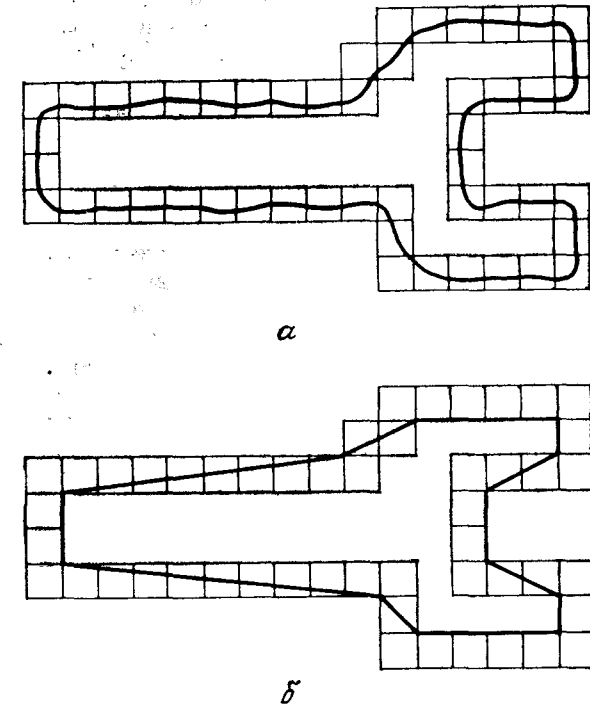
Рис. 8.30. Граница объекта, заключенная в элементы (а), и многоугольник минимального периметра (б).
