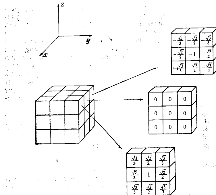
Рис. 8.44. Оператор размерностью 3 \times 3 \times 3 для вычисления составляющей градиента G_x [324].
