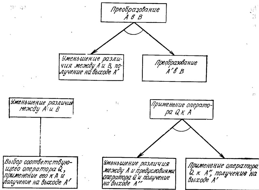
Рис. 10.11. Методы анализа конечных значений.
