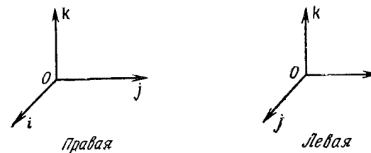
Рис. А.4. Декартова система координат.
