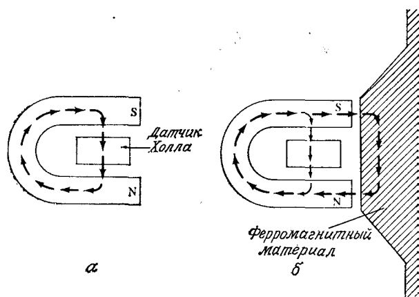
Рис. 6.10. Работа датчика Холла (а), снабженного постоянным магнитом (б).
