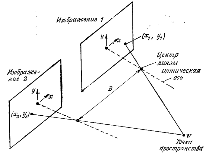
Рис. 7.17. Схема получения стереозображения.
