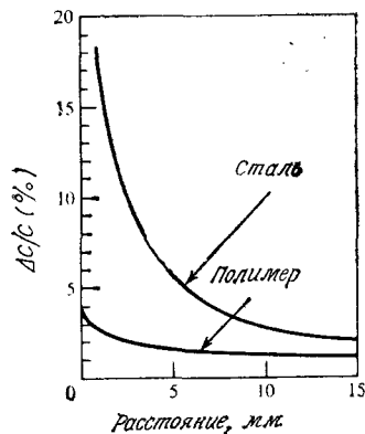
Рис. 6.13. Зависимость процентного изменения емкости датчика в ближней зоне от расстояния [38].
