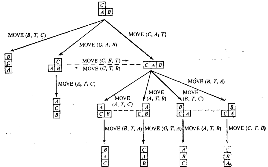
Рис. 10.2. Граф поиска в пространстве состояний.
